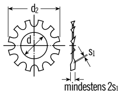
Form A außengezahnt
