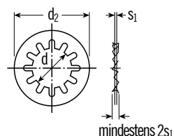
Form J innengezahnt
