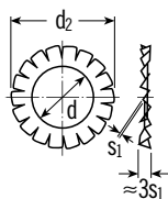
Form A außengezahnt
