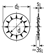
Form J innengezahnt
