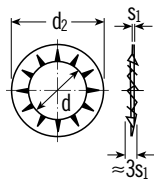
Form J innengezahnt
