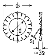
Form A außengezahnt
