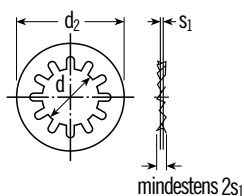
Form J innengezahnt
